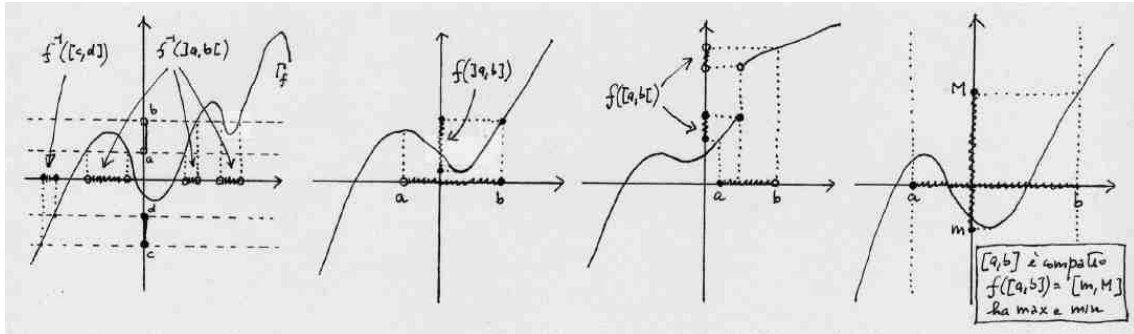
Figura 3.6: Antiimmagini di intervalli tramite funzioni continue; l'immagine di un intervallo tramite una funzione continua è un intervallo; l'immagine di un intervallo tramite una funzione discontinua può non essere un intervallo; il teorema di Weierstrass.
