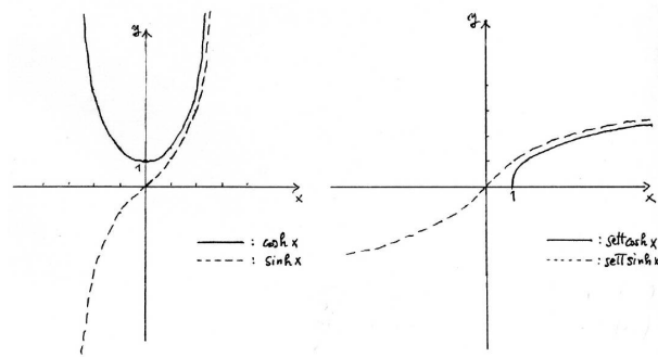
Figura 3.8: Grafici del seno iperbolico \sinh , del coseno iperbolico \cosh e delle loro inverse \text{setth sinh} e \text{setth cosh} .
