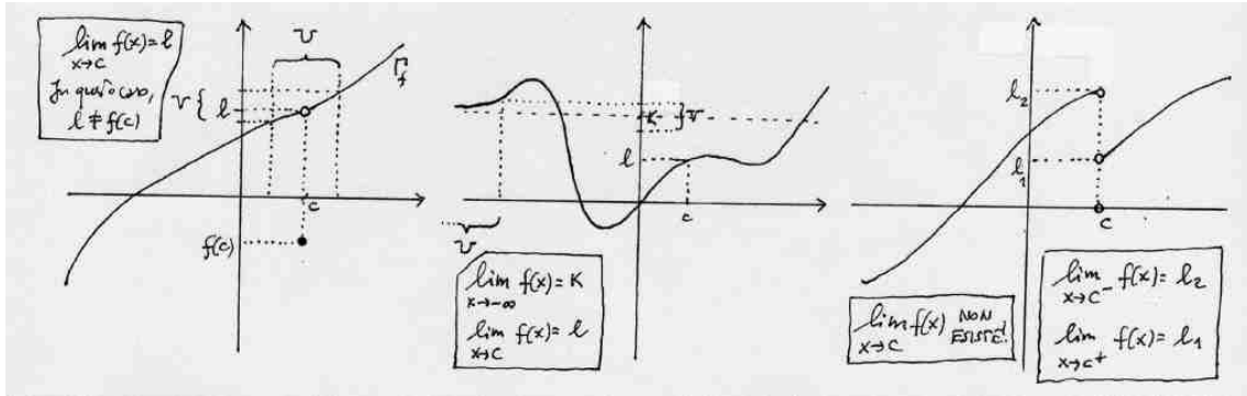
Figura 3.4: Esempi visivi di limiti; limite sinistro e limite destro.
