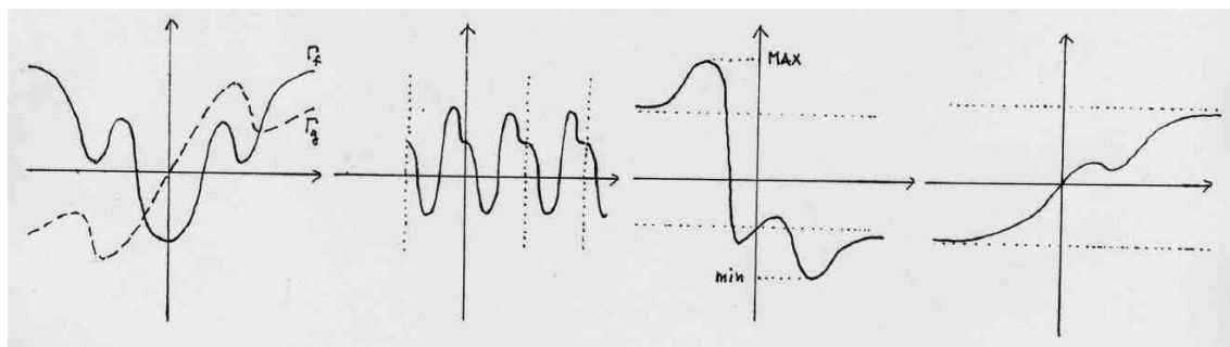
Figura 3.2: Grafico di una funzione pari f e dispari g ; grafico di una funzione periodica; grafico di una funzione limitata con massimo e minimo; grafico di una funzione limitata priva sia di massimo che di minimo.
