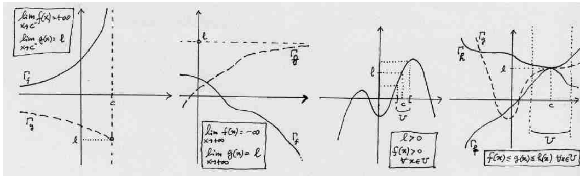
Figura 3.5: Limiti di funzioni monotone in c \in \mathbb{R} e in +\infty ; permanenza del segno; i due carabinieri.
