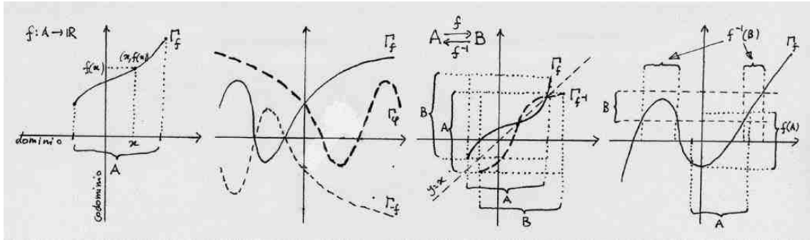
Figura 3.1: Grafico di una funzione; grafici della funzione opposta e speculare; grafico della funzione inversa; immagine e antiimmagine sul grafico.
