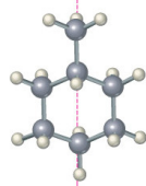
Metilcicloesano (achirale)
