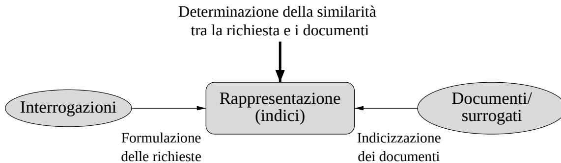
Figura 2: Architettura funzionale di un sistema di IR
