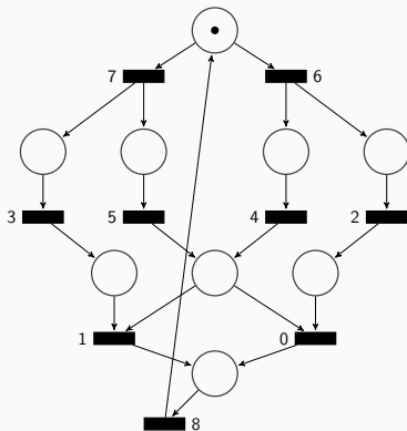
Rete di Petri risultante con l'unione delle pre-regioni
