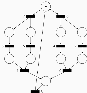
Rete di Petri risultante senza l'unione delle pre-regioni
