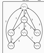
Grafo di raggiungibilità
