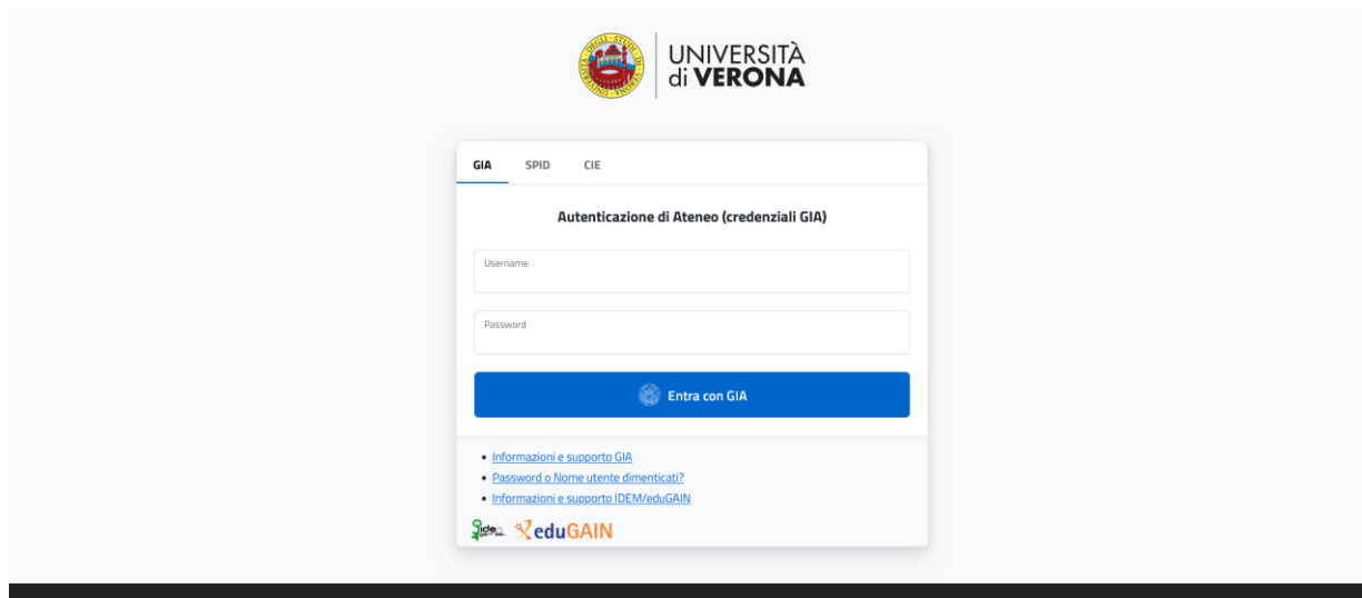
Figura 1: Autenticazione
