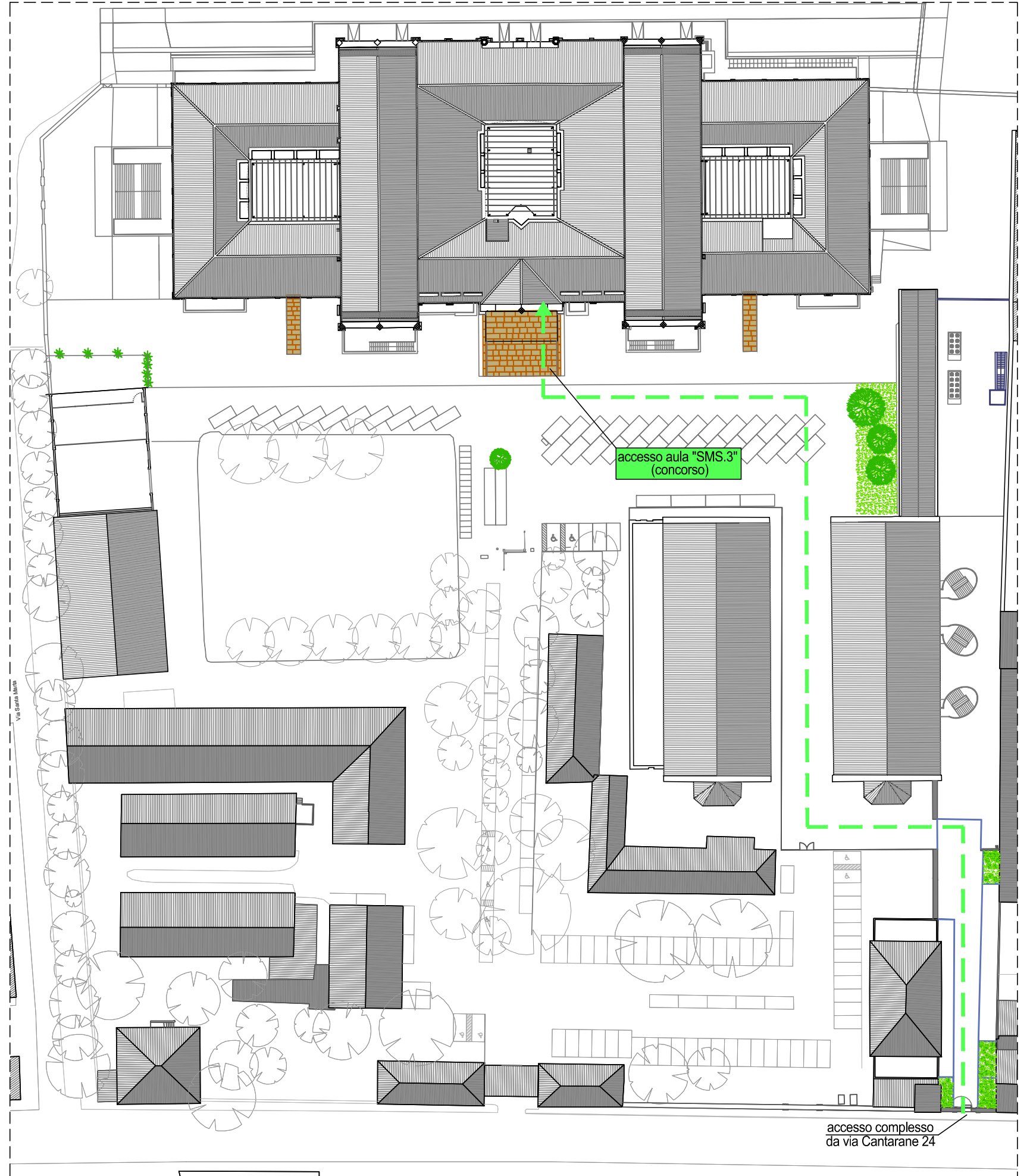
PLANIMETRIA GENERALE
